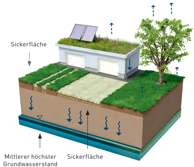
Abbildung 28: Flächenversickerung
