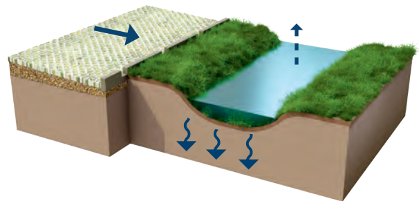
Rigolenversickerung
